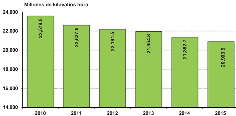
Gráfica 37: Generación de energía eléctrica Puerto Rico, Años fiscales 2010 – 2015
