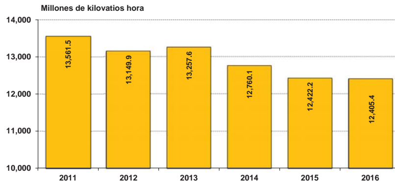
Gráfica 38: Generación de energía eléctrica Puerto Rico, Años fiscales 2011 - 2016 Acumulado julio a enero
